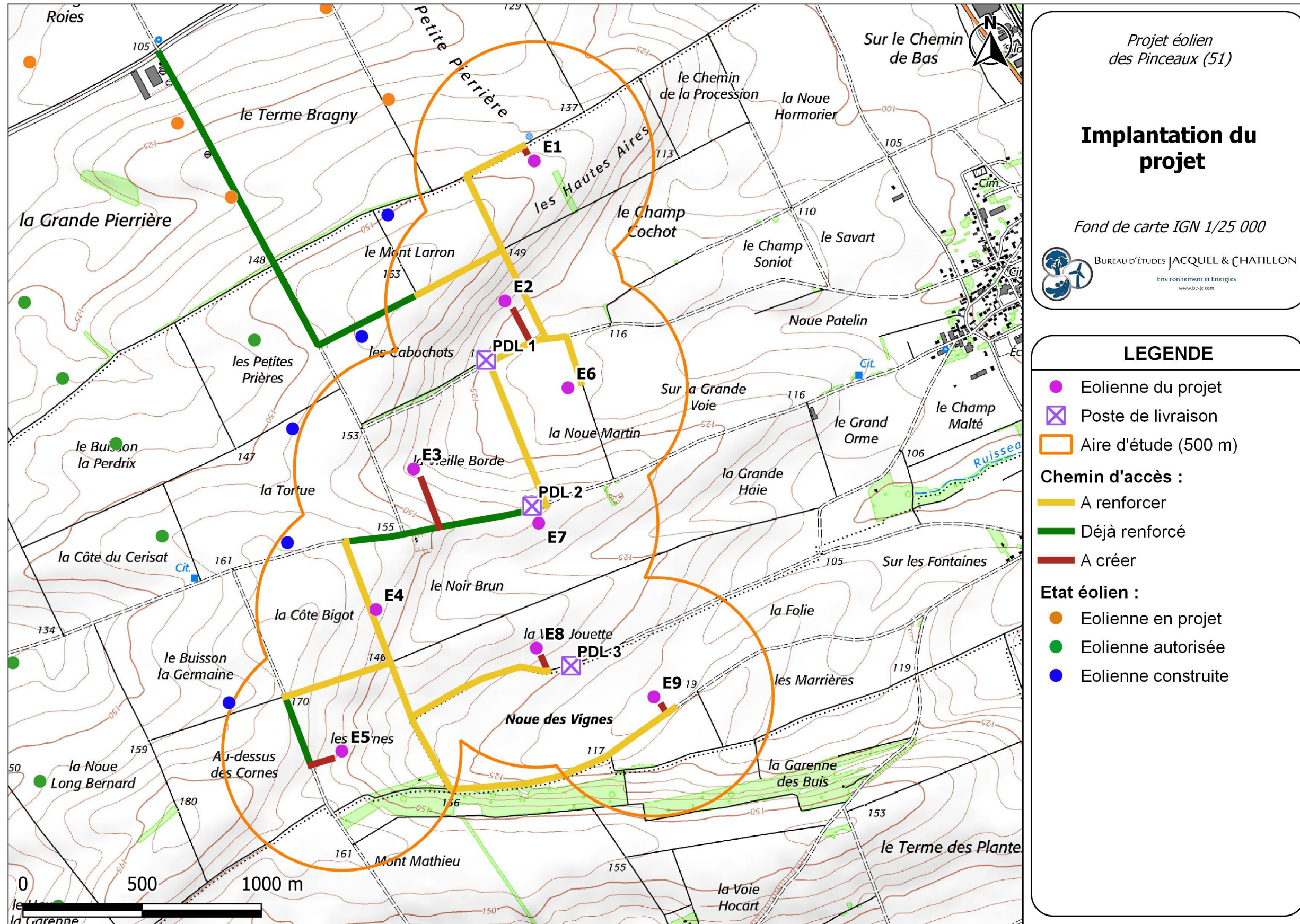
Carte 25 : Configuration de l'installation (Source : BE Jacquél et Chatillon)
